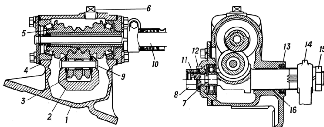
Hình 10.14. Cơ cấu kiểu trục vít-con lăn
