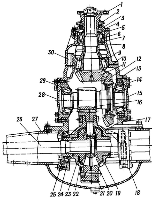
Hình 10.11 Truyền lực chính kép ZIL-130
