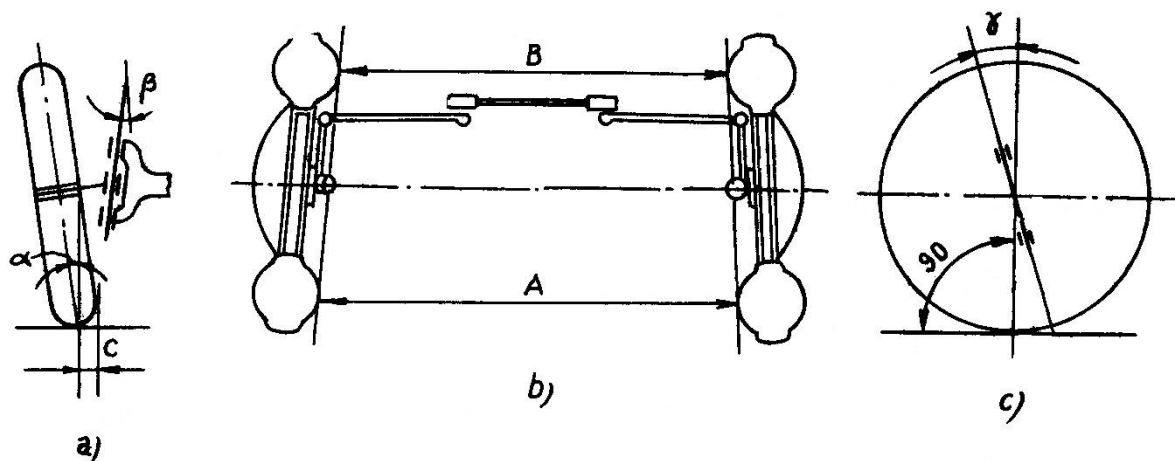
Hình 10.13. Góc đặt bánh xe
