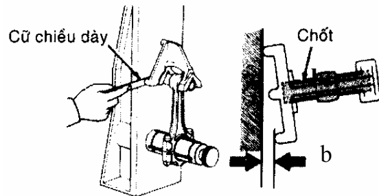
(B) Thanh truyền bị xoắn
