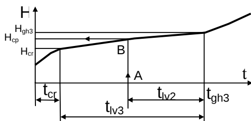
Hình 6.3 Cách xác định thời gian tiếp tục làm việc của chi tiết
