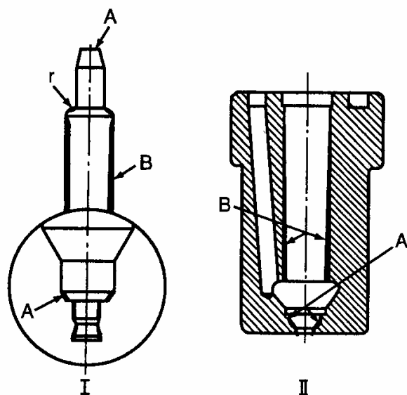
Hình 9.16 Mòn thân kim phun và đế I. Mòn phần côn kim A và chốt B II. Mòn phần côn để kim A và lỗ chốt B
