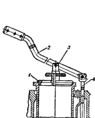
Hình 7.3. Vam ép xi lanh ướt 1-Bích ép; 2-tay đòn ép; 3-đầu lắp bích ép; 4-vít bắt đồ gá ép lên thân
