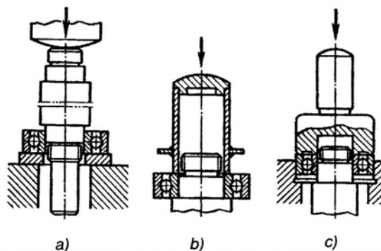
Hình 7.21 Lắp vòng bi a-lắp vòng bi vào trực; b-lắp vòng bi vào trực với đầu ép; c-Lắp vòng bi vào lỗ và trực với đầu ép
