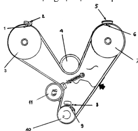
Hình 7.15 Lắp dây đai 1-2, 5-6- dấu trên các bánh đai trục cam và nắp máy; 8-9-dấu trên bánh đai trục khuỷu và thân máy; 4-bánh đai bơm nước; 3-7-bánh đai trục cam;
