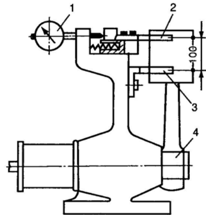
Hình 7.9 Đồ gá kiểm tra độ thẳng nhóm piston-thanh truyền
