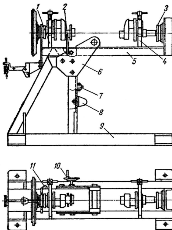
Hình 7.6 Giá lắp trục khuỷu và bánh đà
