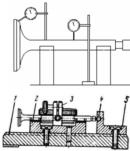
Hình 6.11. Sơ đồ và dụng cụ kiểm tra cong xu páp 1 _ giá dụng cụ; 2 _ khối V; 3 _ giá đồng hồ so; 4 _ bi tì; 5 _ tấm cữ; 6,7 _ các đồng hồ so
