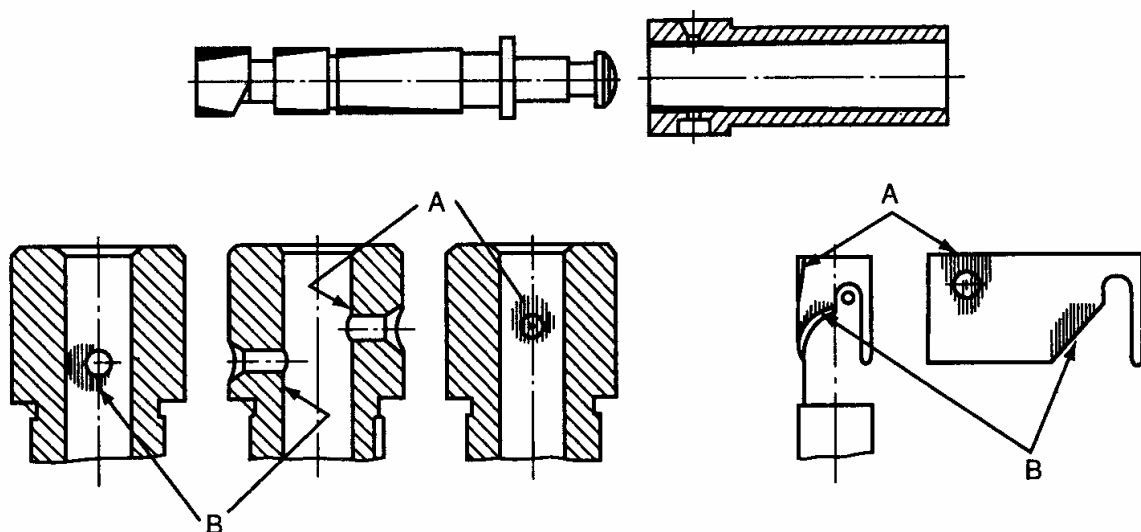
Hình 9.13 Mòn xi lanh và piston bơm cao áp
