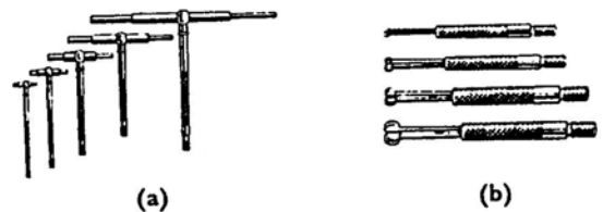
Hình 5.31 Dụng cụ đo đường kính những lỗ nhỏ
