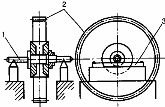
Hình 6.24 Kiểm tra cân bằng trên dao lăn
