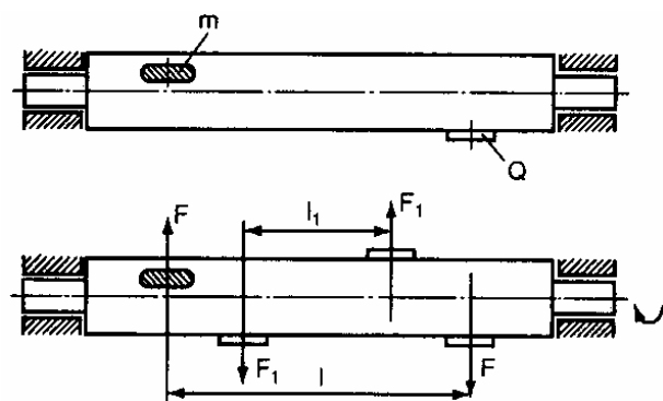
Hình 6.26 Sơ đồ nguyên tắc cân bằng động chi tiết trục trên 2 mặt phẳng chọn trước
