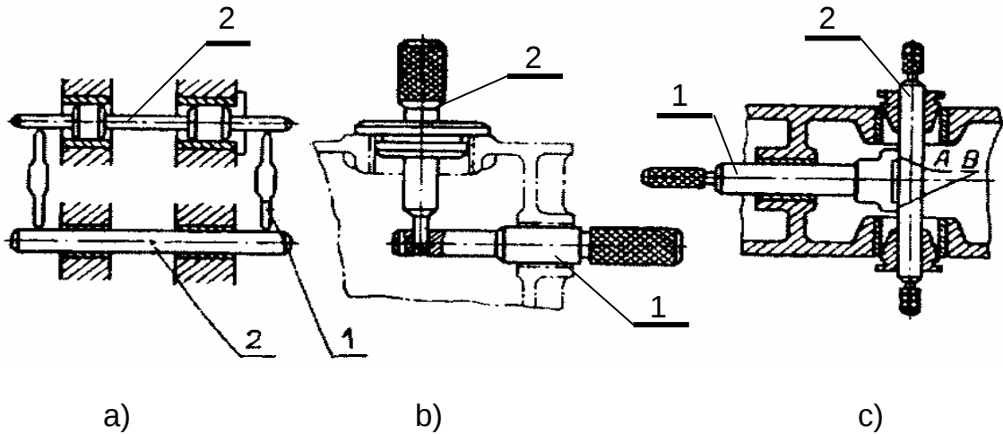
Hình 6.16 Kiểm tra độ song song và vuông góc giữa hai hàng lỗ
