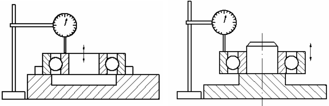
Hình 6.19 Kiểm tra rơ dọc trục của vòng bi
