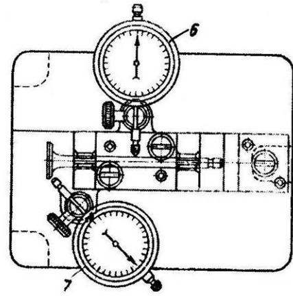
Hình 6.11. Sơ đồ và dụng cụ kiểm tra cong xu páp 1 _ giá dụng cụ; 2 _ khối V; 3 _ giá đồng hồ so; 4 _ bi tì; 5 _ tấm cữ; 6,7 _ các đồng hồ so
