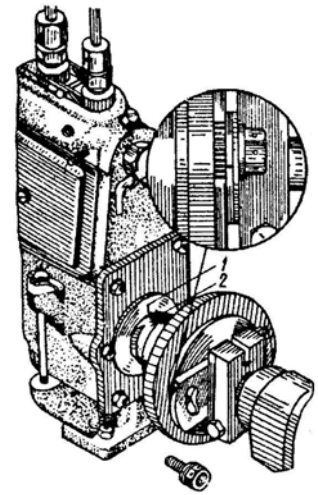
Hình 7.18 Lắp bơm cao áp 1-dấu lắp trên vỏ bơm; 2-dấu trên khớp nối bơm
