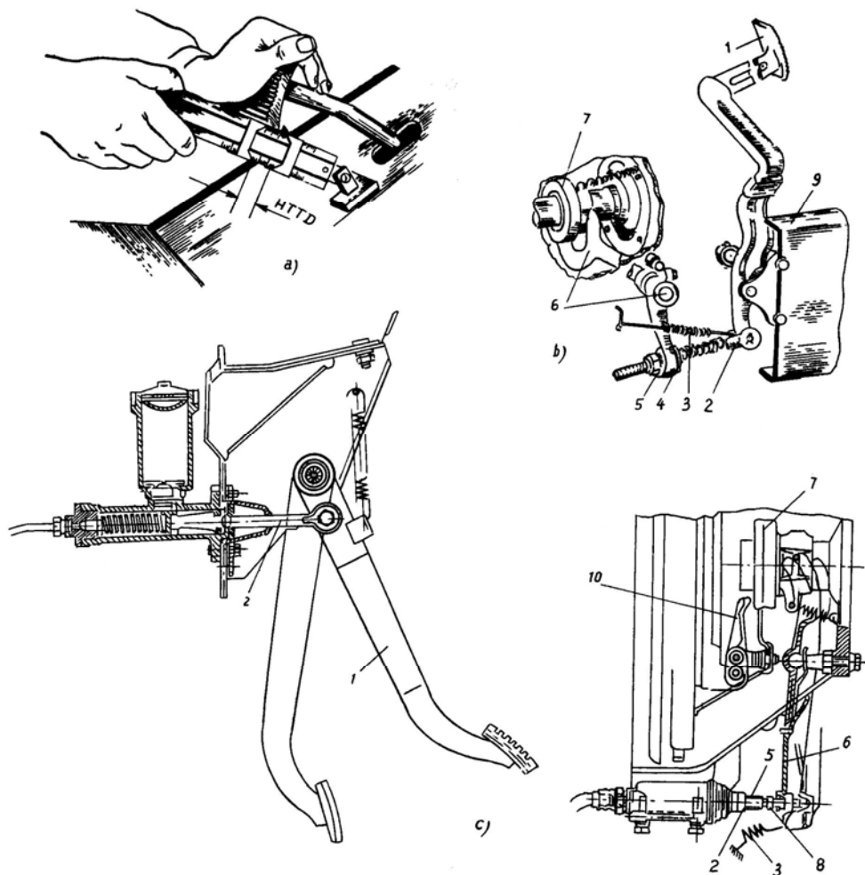
Hình 10. 5. Kiểm tra và điều chỉnh hành trình tự do của bàn đạp ly hợp
