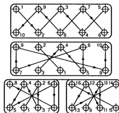
Hình 7.14 Thứ tự siết nắp máy
