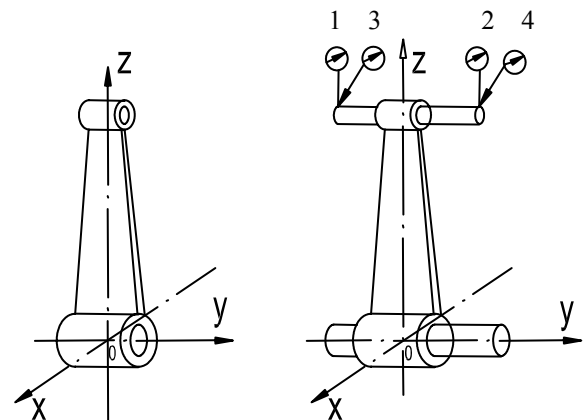
Hình 6.12 Kiểm tra cong, xoắn thanh truyền bằng đồng hồ so
