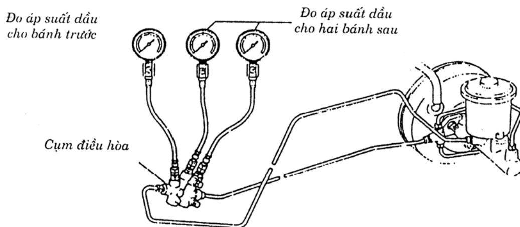
Hình 10.46. Chẩn đoán sự làm việc của bộ điều hòa lực phanh
