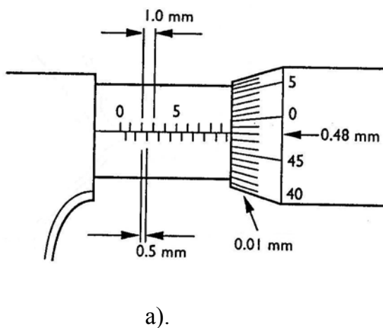
Hình 5. 26 Cách đọc kích thước trên Panme
