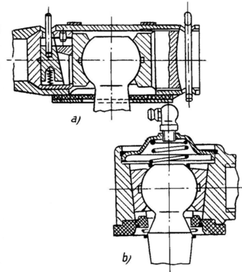
Hình 10.31. Loại khớp cầu tự động điều chỉnh độ rơ trong quá trình làm việc
