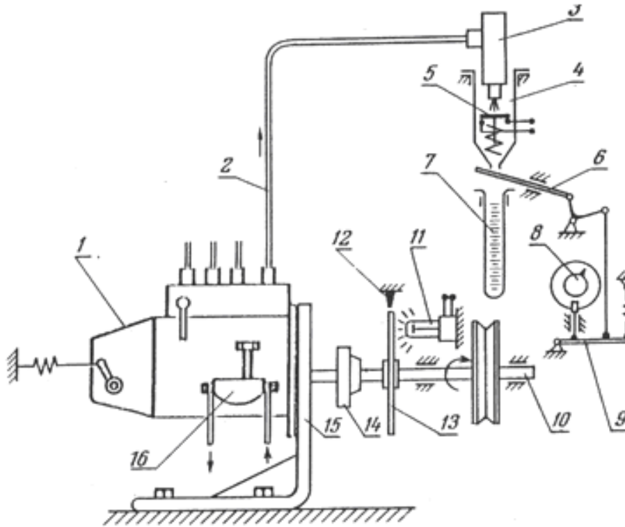
Hình 9.21 Sơ đồ dẫn động bằng thử bơm cao áp
