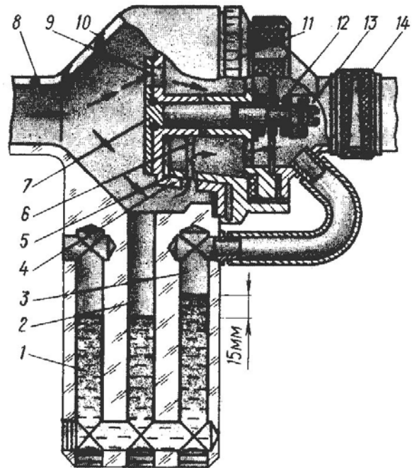
Hình 9.3 Dụng cụ đo lọt khí các te
