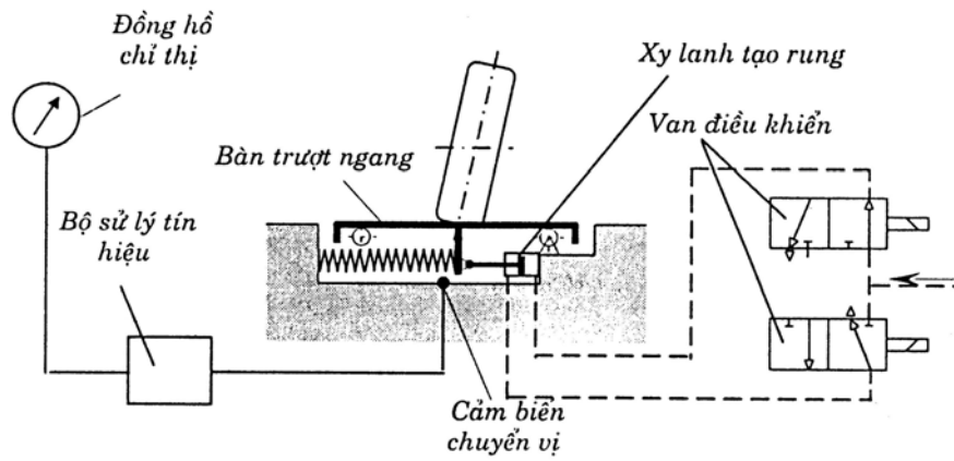
Hình 10.26. Sơ đồ nguyên lý của thiết bị đo độ trượt ngang động
