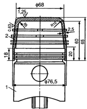
Hình 7.10 Chup lắp séc măng 1-piston; 2-chup lắp séc măng
