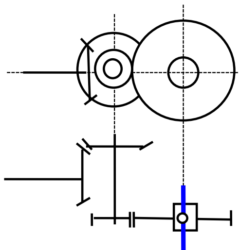
Hình 10.9 Truyền lực chính kép kiểu tập trung
