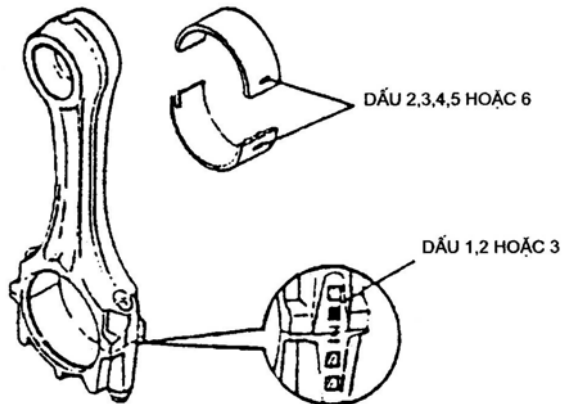
Hình 7. 25 Dấu đánh trên thân, trên trục khuỷu và thanh truyền để chọn lắp bạc
