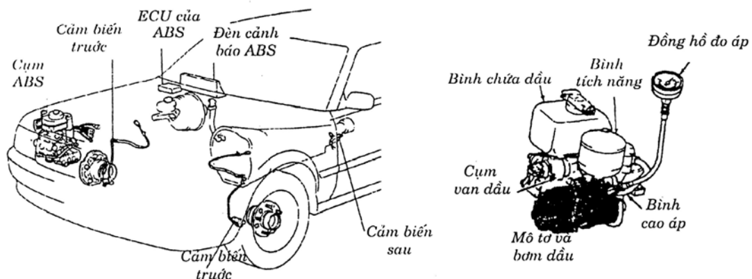
Hình 10.50. Kiểm tra áp suất trên bình tích năng của ABS
