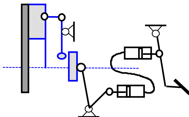
Hình 10.4. Sơ đồ li hợp dẫn động thủy lực
