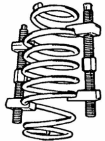
Hình 5.21 Dụng cụ ép lò xo
