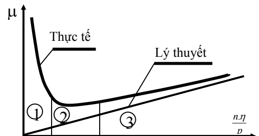
Hình 1.8. Ảnh hưởng của n, \eta, p đến hệ số ma sát.
