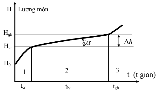
Hình 3.1. Đồ thị mài mòn chi tiết
