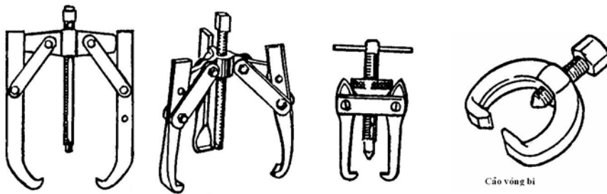
Hình 5.20. Các loại cảo bánh răng, bánh đai, vòng bi.
