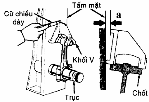
(A) Thanh truyền bị cong
