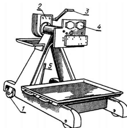
Hình 7.2. Giá lắp động cơ nhẹ 1-bánh xe; 2-hộp trục vít; 3-tay quay; 4-bích lắp động cơ; 5-tay hãm động cơ
