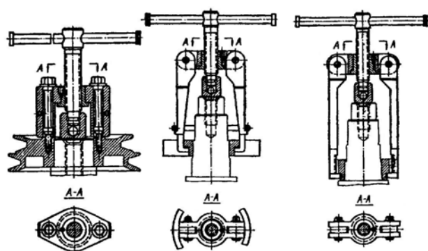
Hình 7.20 Các loại vam a-vam tháo puli đầu trực khuỷu; b-vam tháo vành chặn dầu; c-vam tháo bánh răng.
