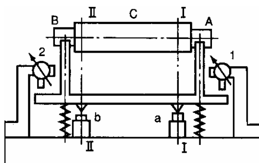
Hình 6.27 Nguyên lý thiết bị cân bằng động trên 2 mặt phẳng chọn trước 1,2 cảm biến biên độ dao động khung a,b các ổ tì; A,B các ổ đỡ trục trục trên khung dao động.
