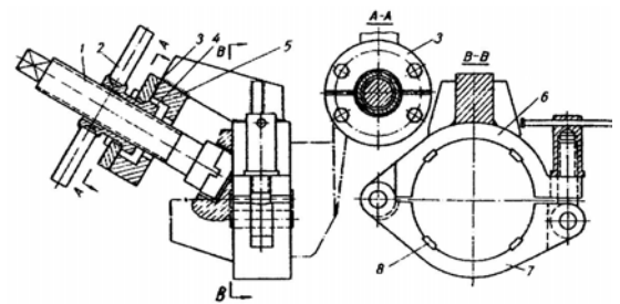
Hình 7.7 Dụng cụ tháo lắp nút dầu trên trực khuỷu
