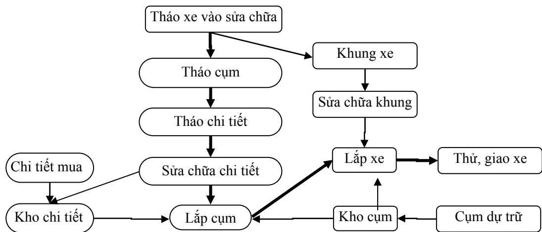
Hình 5.4. Sơ đồ quá trình công nghệ sửa chữa theo phương pháp đổi lẫn
