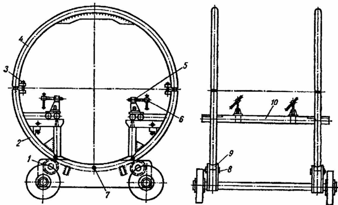
Hình 7.1. Giá lắp động cơ có khối lượng nặng 1-Đế khung; 2-nửa khung dưới; 3-bu lông kẹp; 4-nửa khung trên; 5-giá di động kẹp động cơ; 6-vít kẹp; 7-chốt hãm trục con lăn; 9-con lăn tì; 10-thanh ngang.
