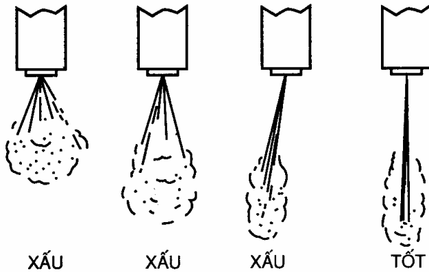
Hình 9.18 Kiểm tra chất lượng chùm tia phun
