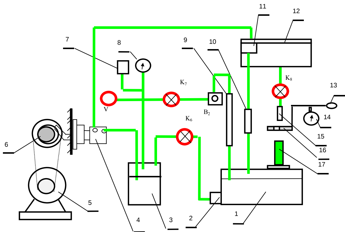
Hình 9.10 Hệ thống kiểm tra bộ chế hoà khí dùng nước trên thiết bị MBKV2
