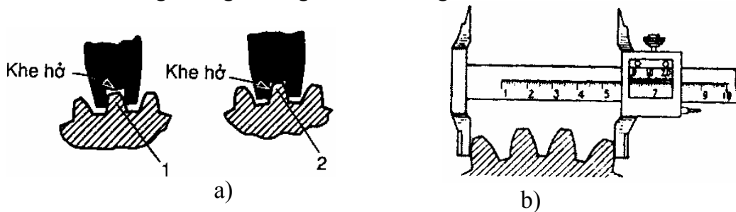
Hình 6.21 Kiểm tra mòn răng bằng dưỡng đo răng (a) và thước cặp (b)
