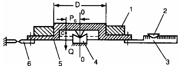
Hình 6.25 Cân bằng tĩnh trên mâm xoay.
