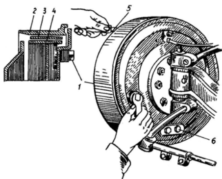
Hình 10.41. Điều chỉnh khe hở giữa má phanh và trống phanh đối với phanh dầu
