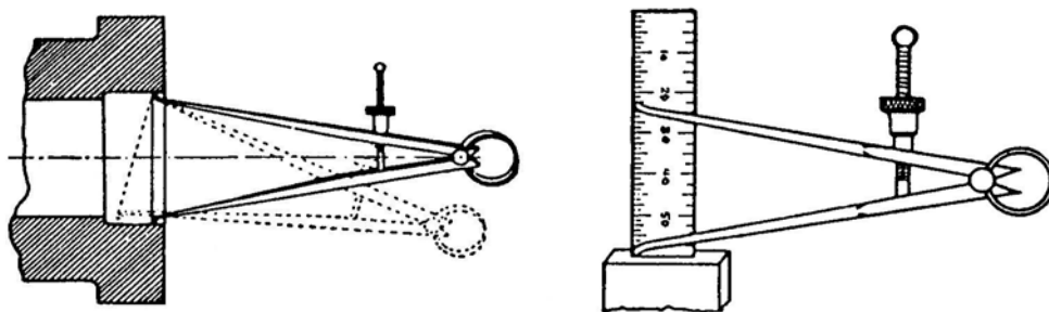
Hình 6.5 Đo kiểm tra chi tiết dạng lỗ
