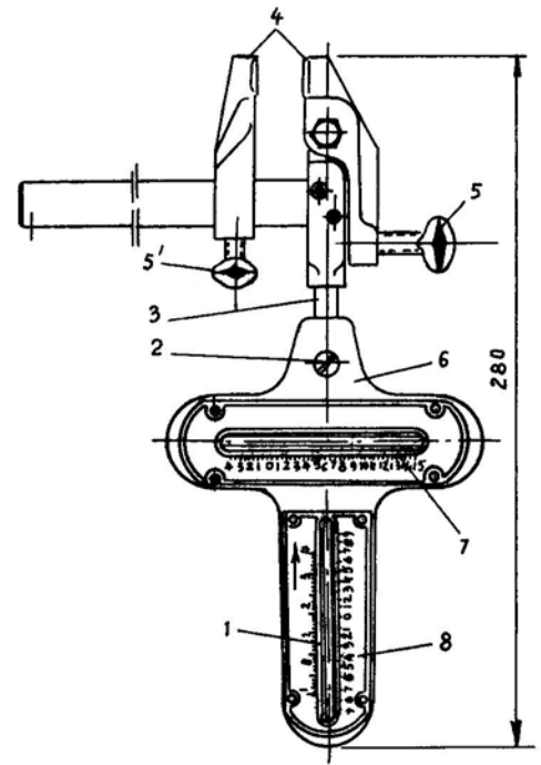
Hình 10.18 Cấu tạo của đồng hồ bọt nước M2142
