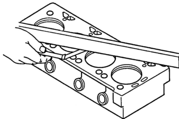
Hình 5.33. Thước kiểm tra mặt phẳng
