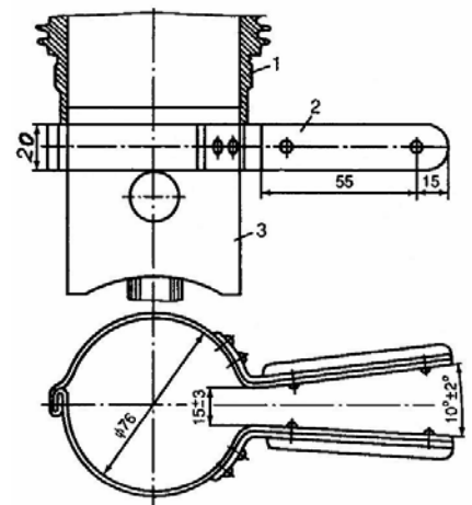
Hình 7.12 Vòng kẹp lắp piston-séc măng vào xi lanh
