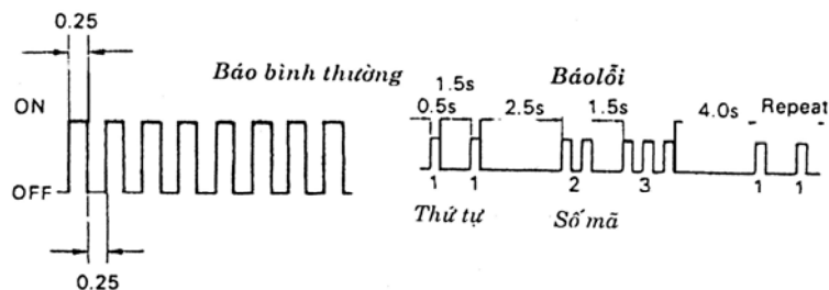
Hình 10.52. Đọc mã
