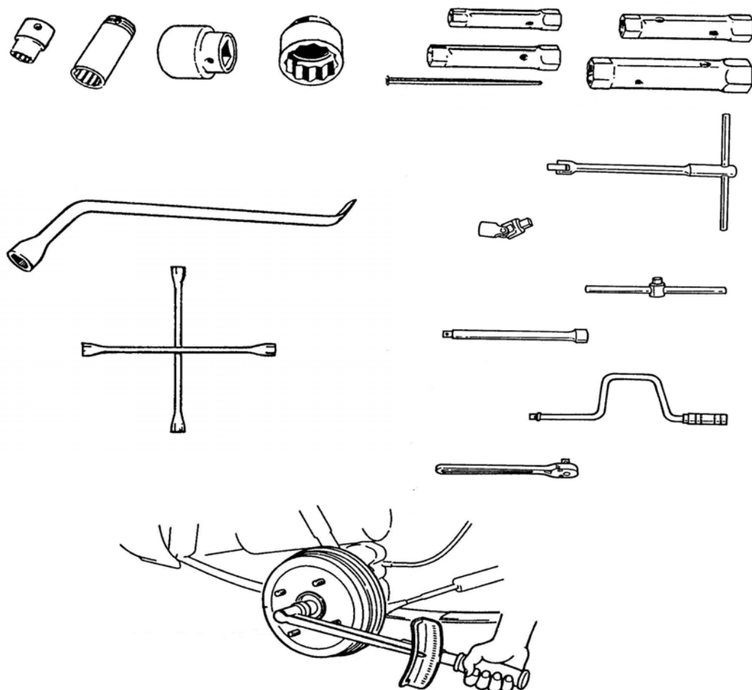
Hình 5.11 Các loại túp và cân siết
