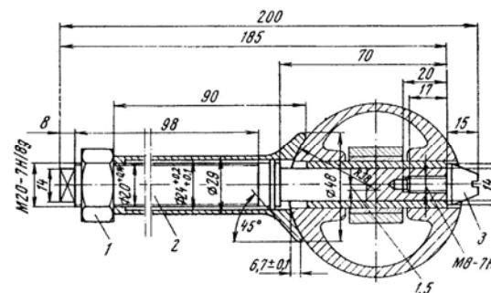
Hình 7.8 Dụng cụ ép chốt piston 1-đai ốc; 2-trực rút; 3-vít hãm
