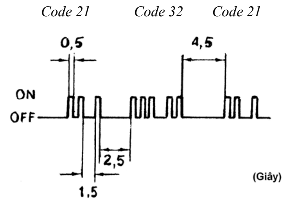
Hình 9.25. Hệ thống có sự cố
