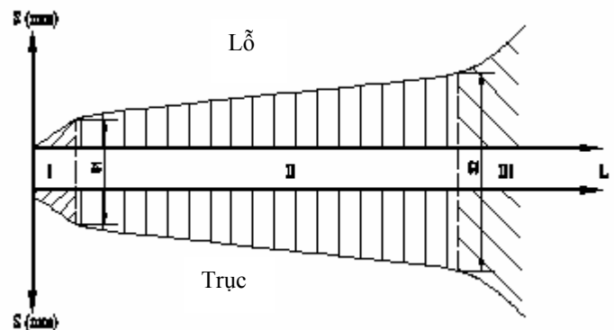
Hình 2.1. Qui luật hao mòn trục, lỗ.
