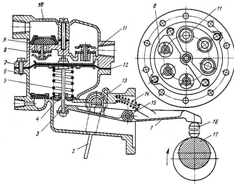
Hình 9.7 Bơm xăng
