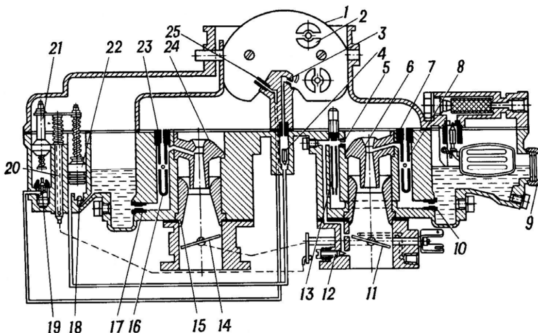
Hình 9.8 Bộ chế hòa khí K-126Г
